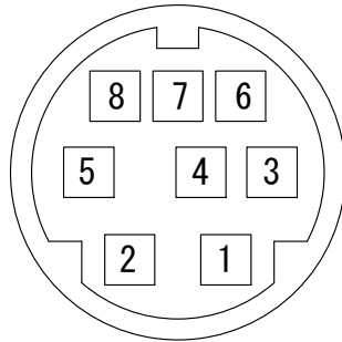
MiniDIN8Pメス座
